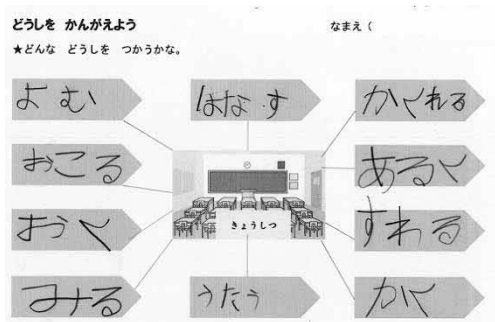
図1 動詞集め
